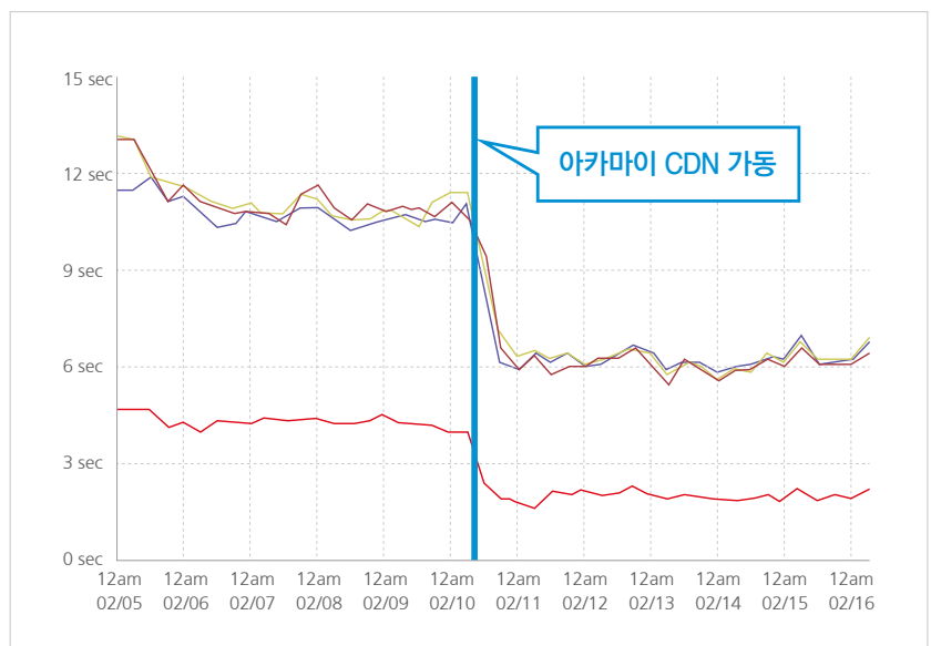
[그림 1] 웹성능 최적화 CDN 사용전/후 페이지 응답시간 변화
