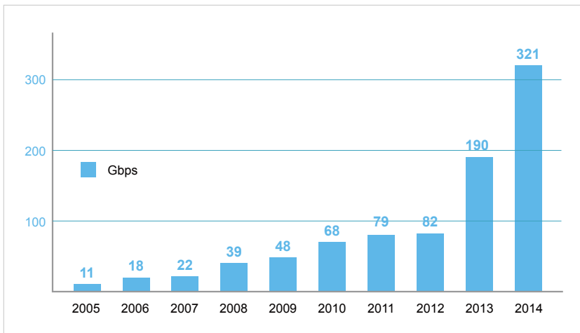
[그림 2] 아카마이 보안 플랫폼에서 관측/처리된 년중 최대 공격 규모 추이
